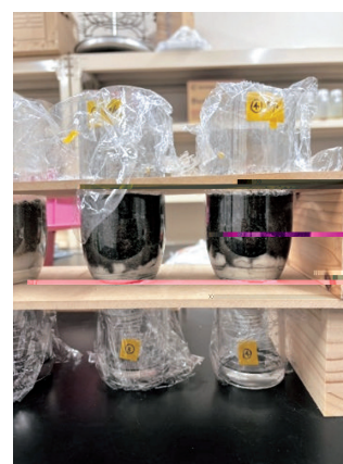
写真1 カラム実験装置の例
